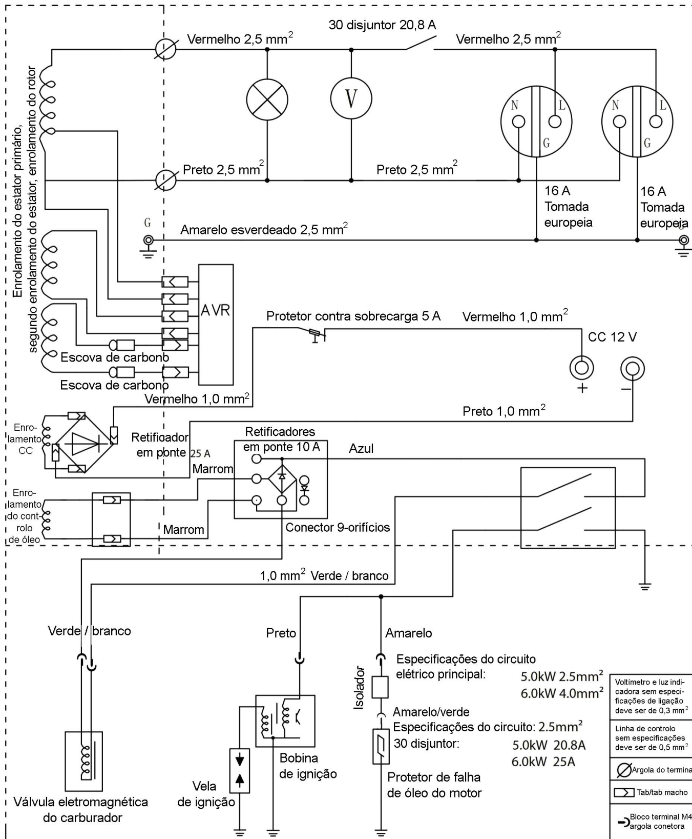
Diagrama Elétrico Esquemático
